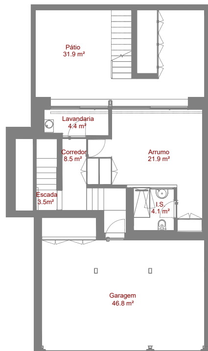
Planta Piso -1
