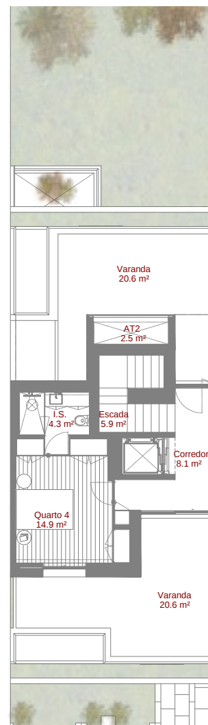
Planta Piso 2
