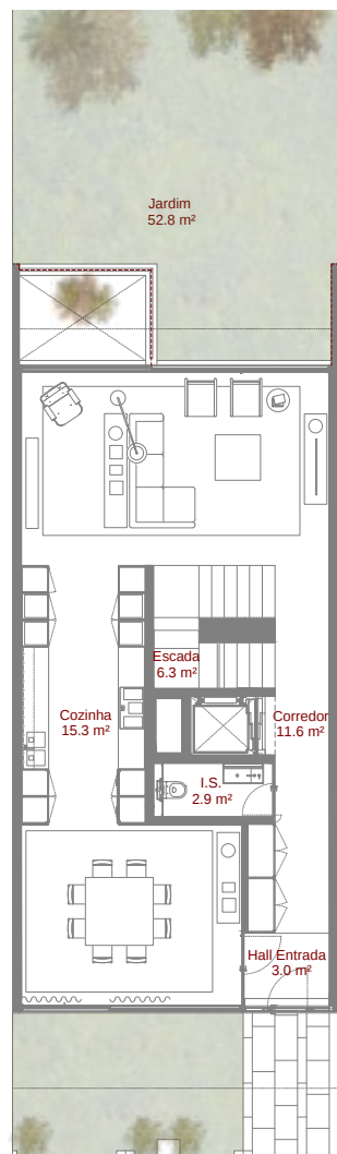
Planta Piso 0
